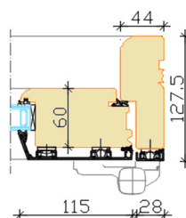
Standard jamb
