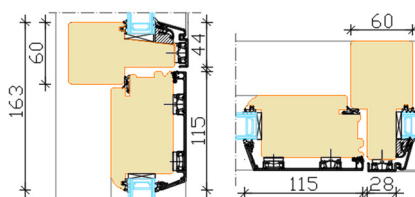
Transom
