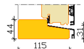
Hardwood door sill
