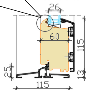
Aluminium door sill
