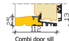
Combi door sill
