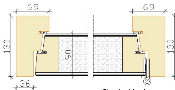
Standard jamb
