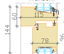
Transom
