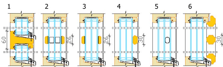
Standard jamb
