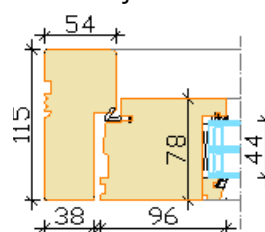
Standard jamb
